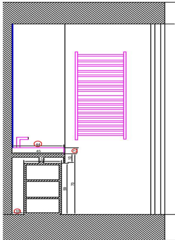
Sezione A.A
