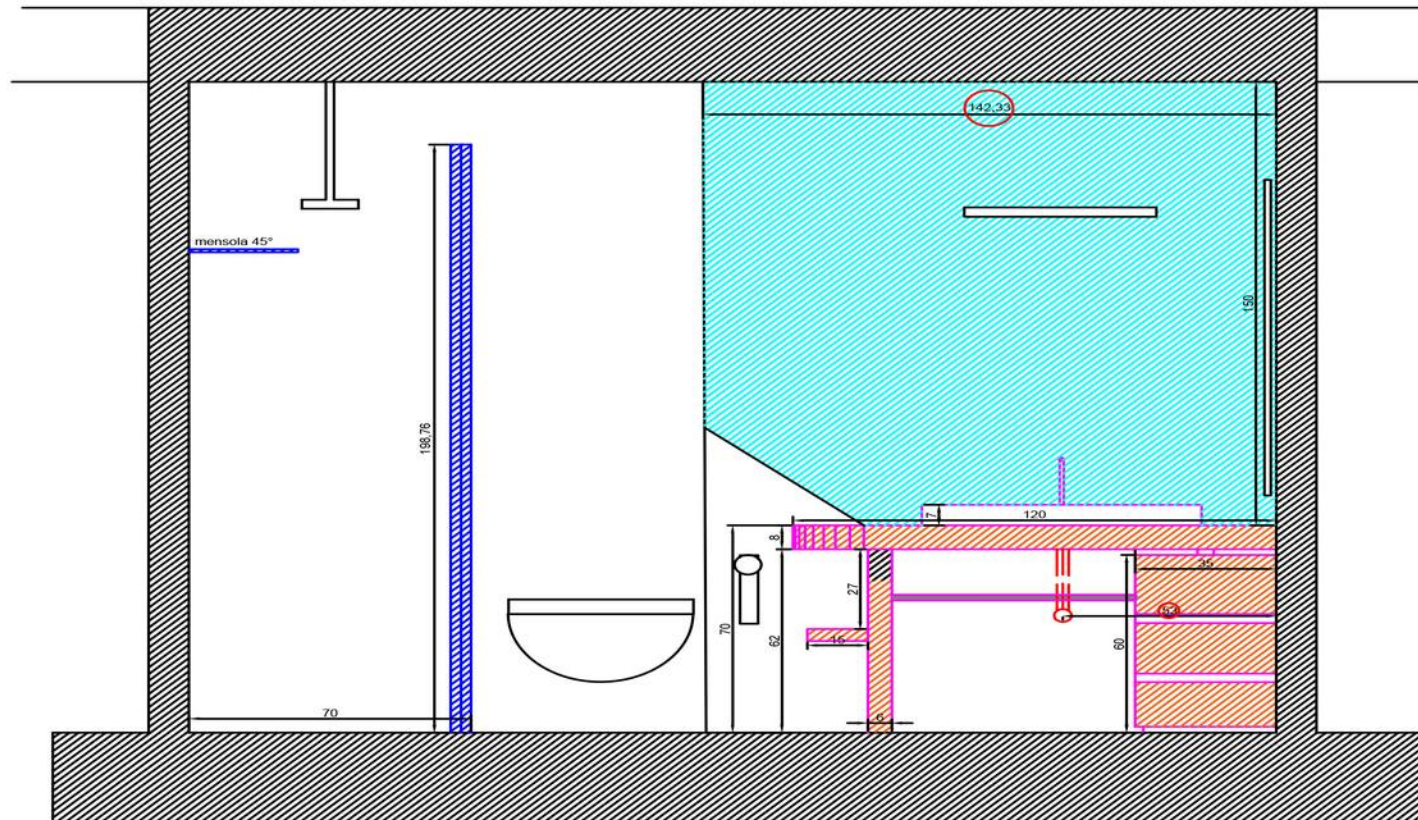
Prospetto bagno
