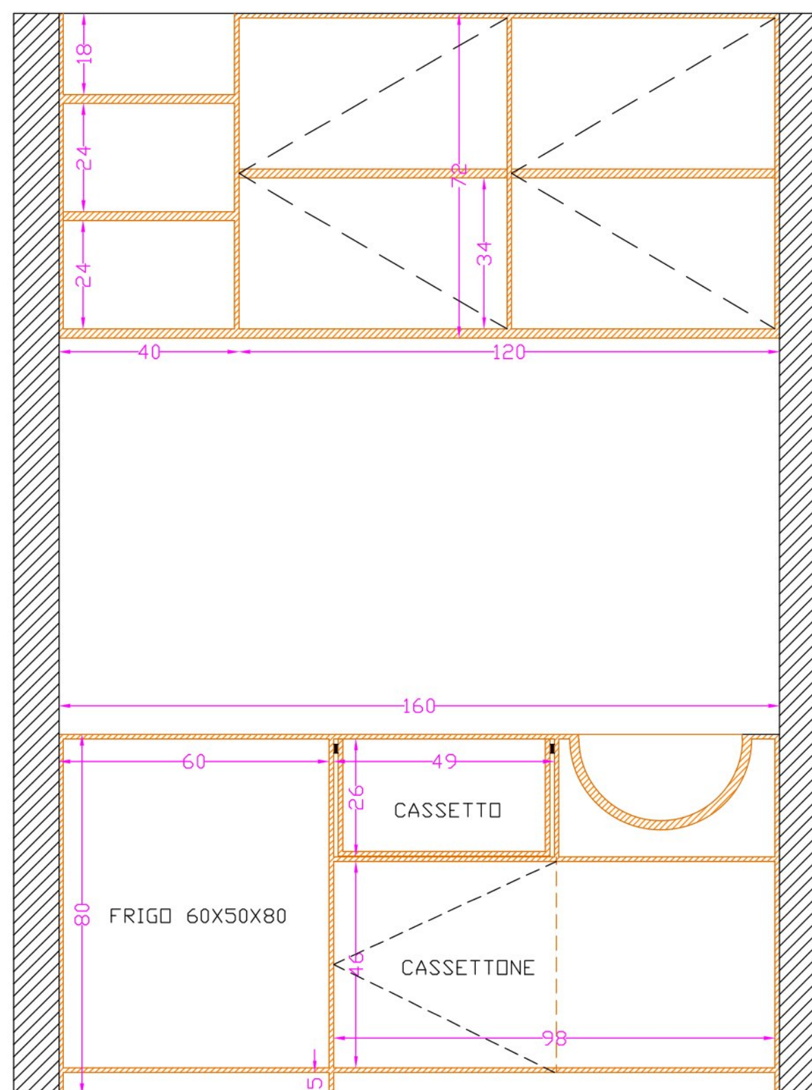
2 CUCINA SEZIONE
