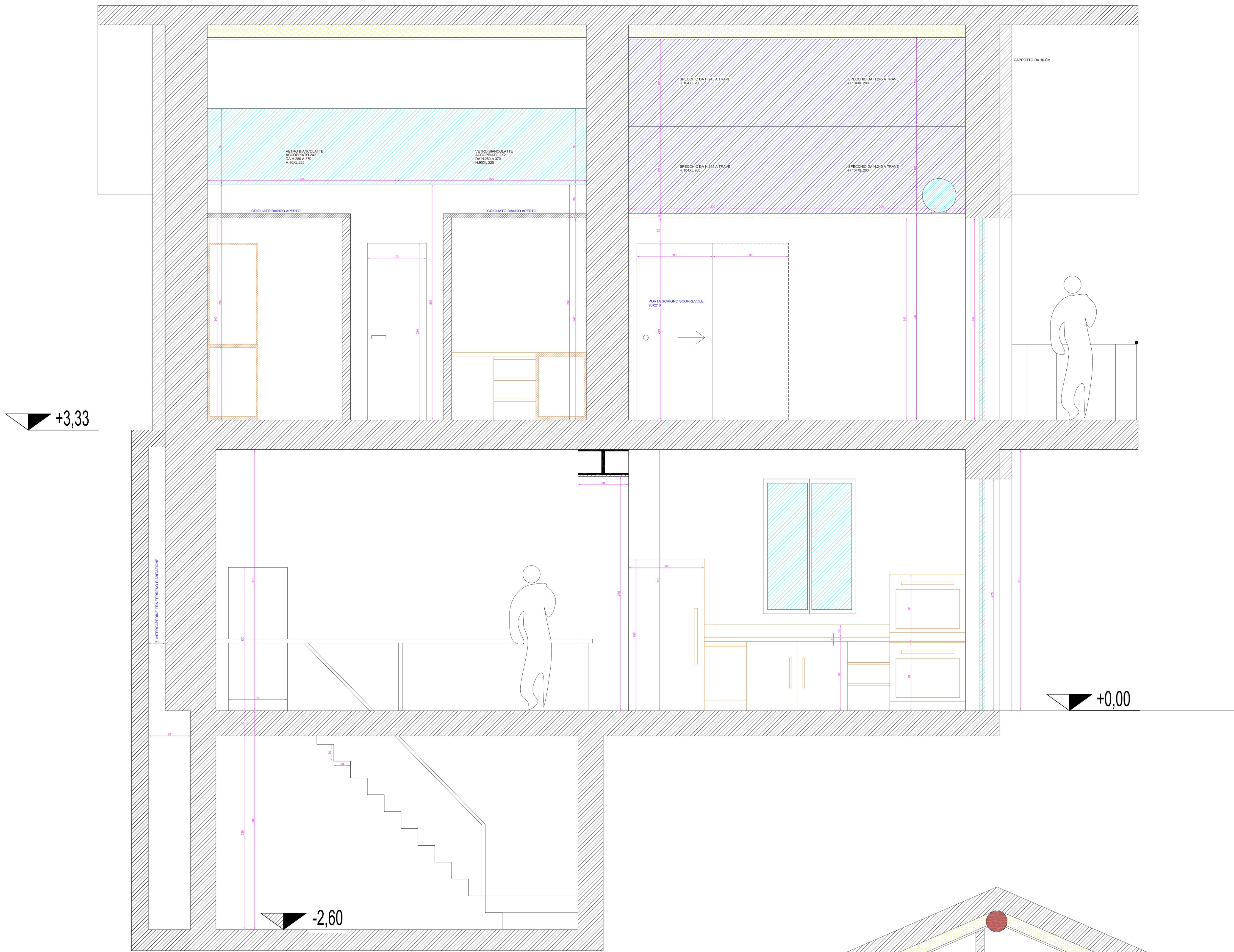
Sezione A-A
