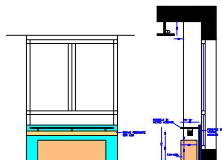
STRUTTURA TIPO REGGINSOLA
